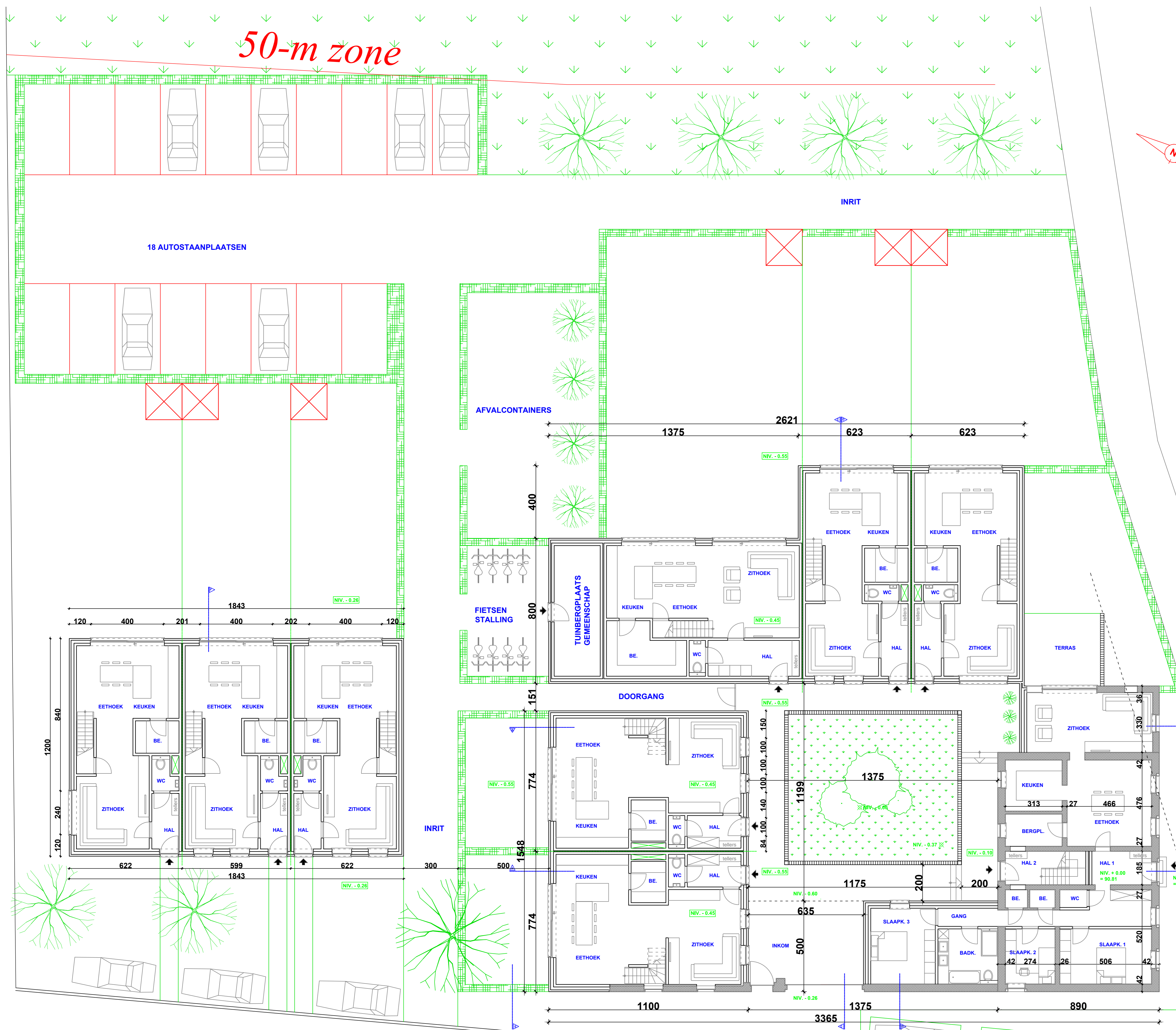
GELIJKVLOERS 1
